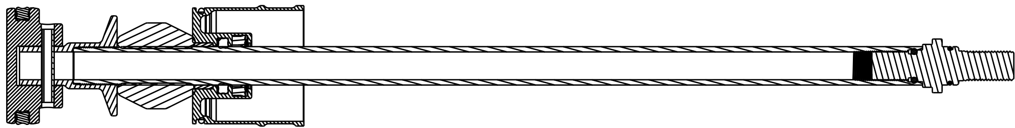
SECTION A-A
